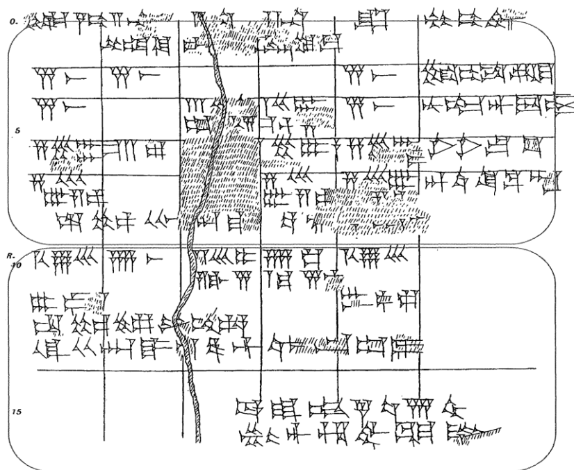
Εικόνα 46: Η πλάκα YBC 4721 ζωγραφισμένη από την E. Robson. 366
