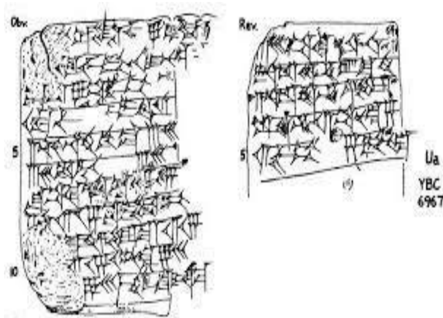
Εικόνα 38: Η πλάκα YBC 6967 281
