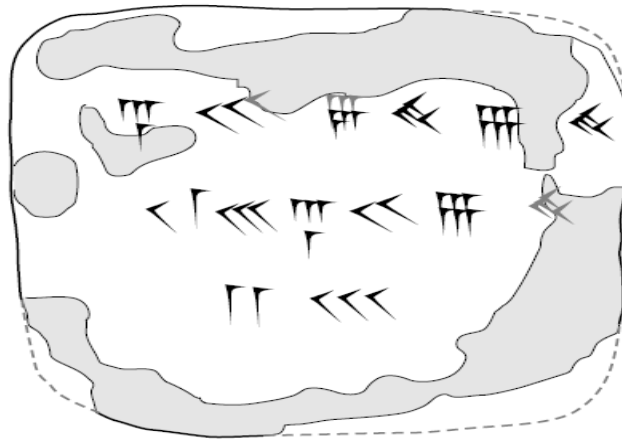
Εικόνα 25: Η πλάκα MS 3871 ζωγραφισμένη από τον Friberg 182
