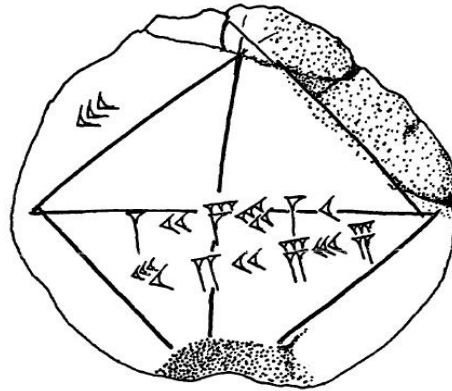
Εικόνα 31: Αναπαράσταση της πλάκας YBC 7289 201
