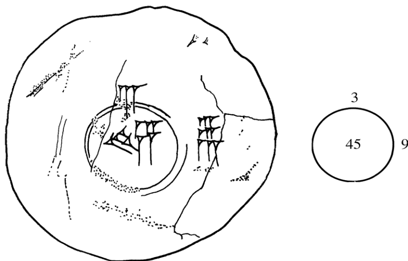
Εικόνα 35: Η πλάκα YBC 7302 ζωγραφισμένη από την E. Robson 223
