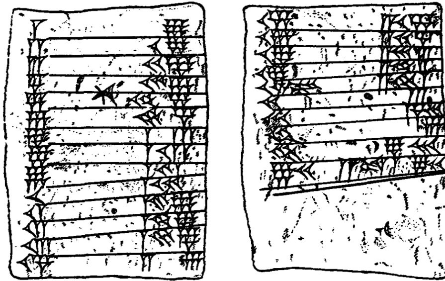
Εικόνα 18: Πίνακας πολλαπλασιασμού για τον αριθμό 9 162
