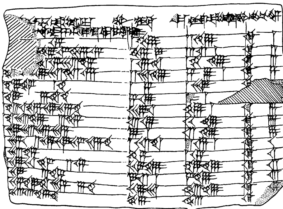
Εικόνα 41: Η πλάκα Plimpton 322 ζωγραφισμένη από την Ε. Robson 314
