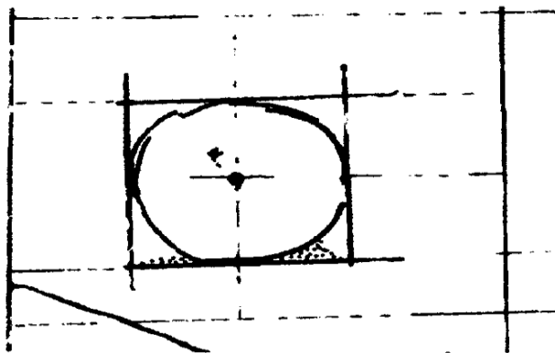
Εικόνα 45: Τμήμα της πλάκας BM 15285 ζωγραφισμένο από την E. Robson 343
